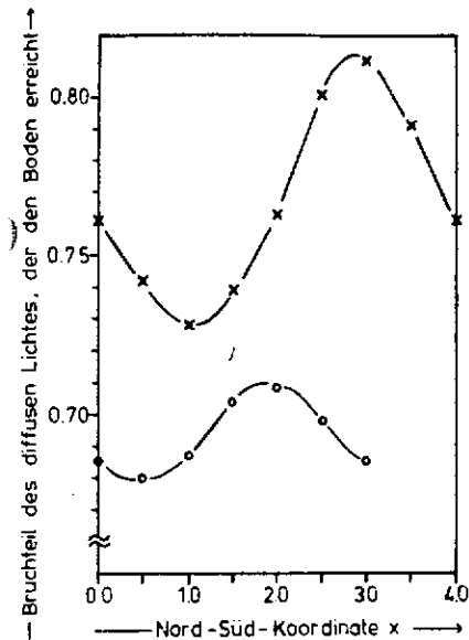
ABB. 4 ABHÄNGIGKEIT DES BRUCHTEILS des diffusen Lichtes, der auf den Boden unter den Kollektoren fällt, von der Nord-Süd-Koordinate
