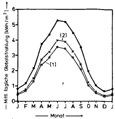
ABB. 6 GLOBALSTRAHLUNG AUF DEM BODEN mit und ohne Kollektoren in Abhängigkeit von der Jahreszeit
